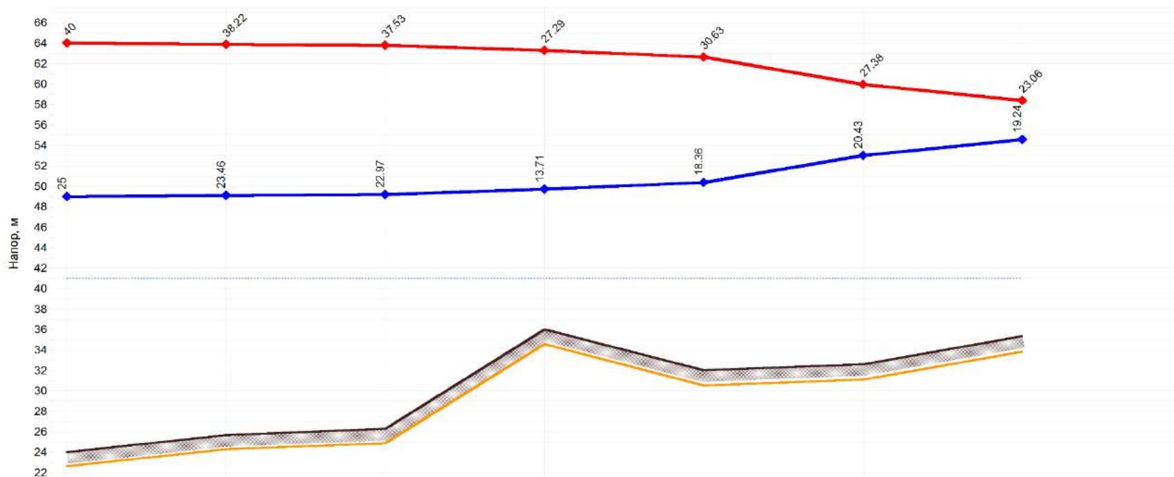
Рисунок 1.3.8.5. - Пьезометрический график от котельной п.Громово до потребителя ж/д №8.
