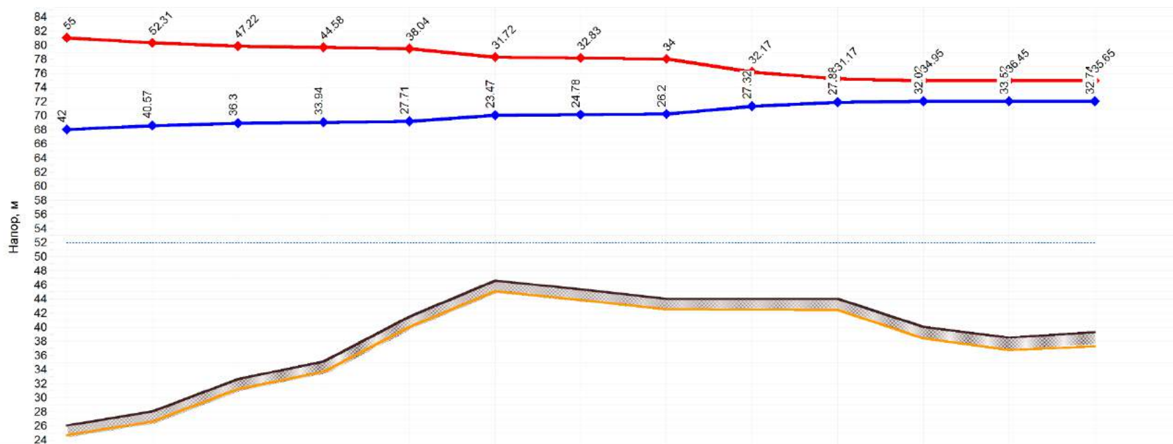
Рисунок 1.3.8.2. - Пьезометрический график от котельной п.Громово до потребителя Д/С.
