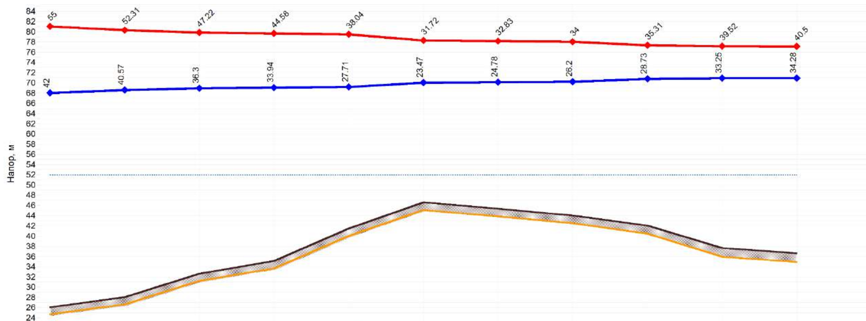
Рисунок 1.3.8.1. - Пьезометрический график от котельной п.Громово до потребителя ж/д №8.
