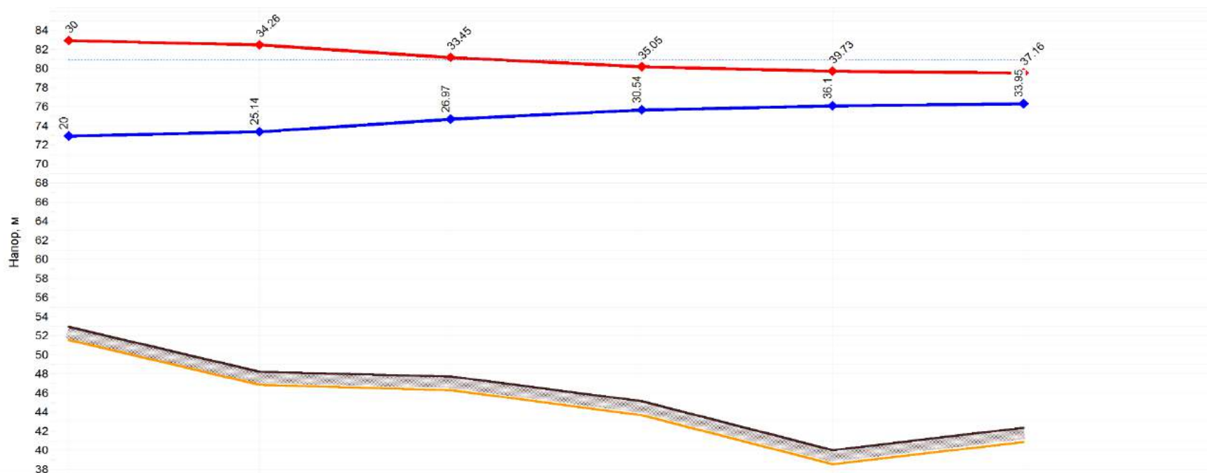
Рисунок 1.3.8.4. - Пьезометрический график от котельной п.ст. Громово до потребителя ж/д №6.
