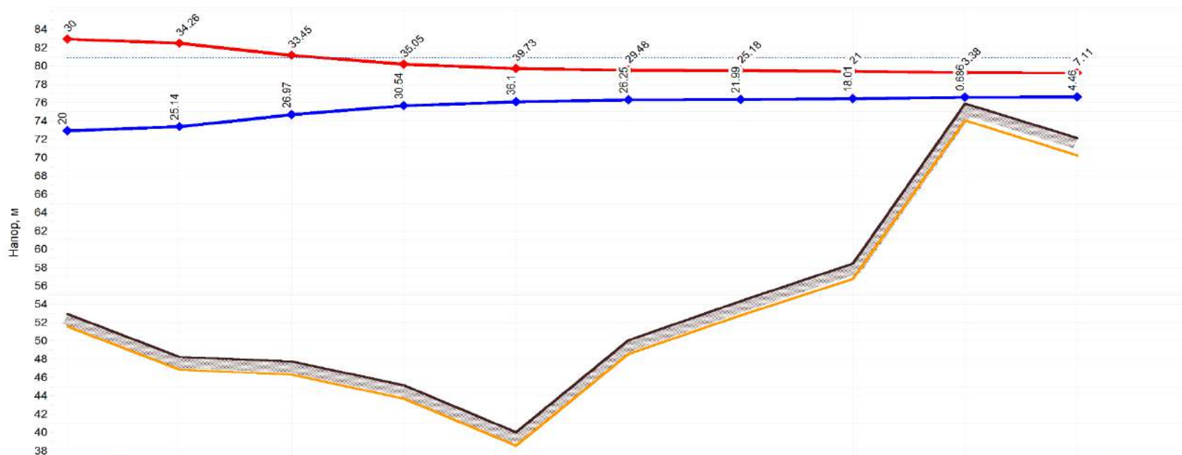
Рисунок 1.3.8.3. - Пьезометрический график от котельной п.ст. Громово до потребителя ж/д №1.
